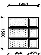
TYPE V3.1 3 stk 158x149 cm
