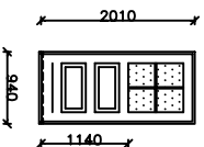
TYPE D1.1 1 stk 94x201 cm INDDØJENDE HH MED 10X50 MM SKINNE ISTEDET FOR BUNDSTYKKE SNYDESPROSSER FOR RUDE
